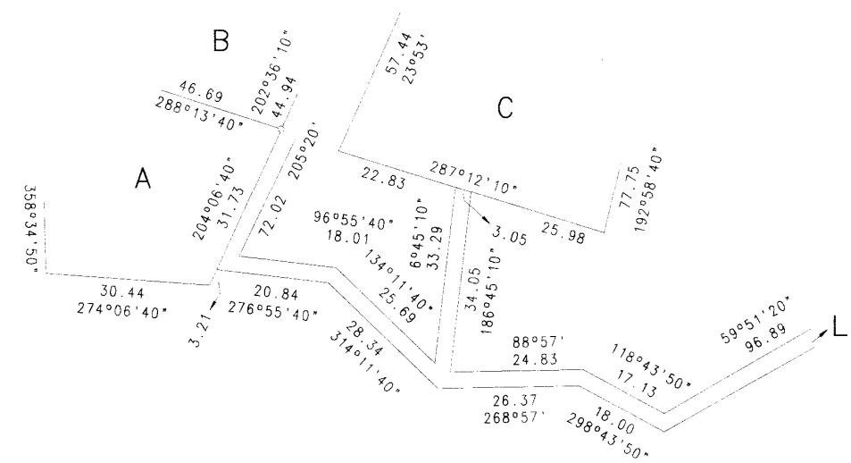
ENLARGEMENT Y NOT TO SCALE
